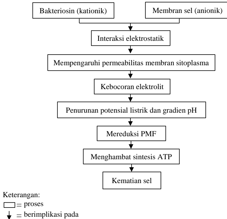
Diagram 1. Mekanisme antibakteri bakteriosin
