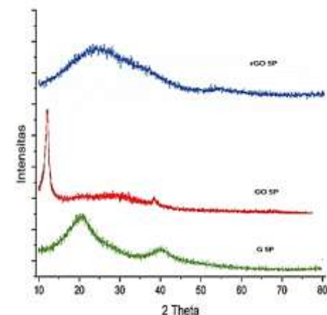
Gambar 2. Difraktogram grafit, GO, dan rGO sekam padi (SP)
